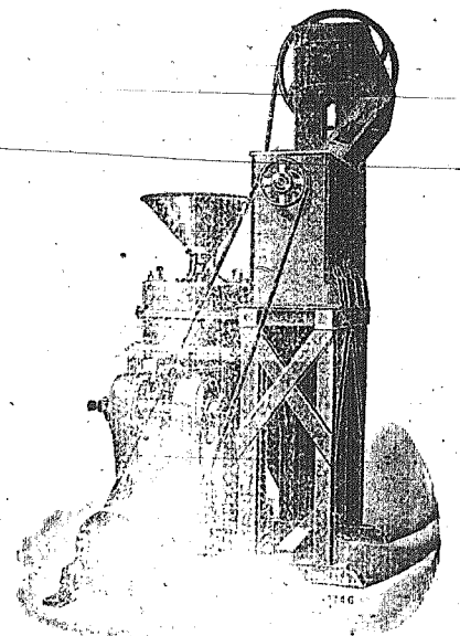
Μύλος, άναβιβαστήριον και σημιδαλίρα συννηνωμένα.
