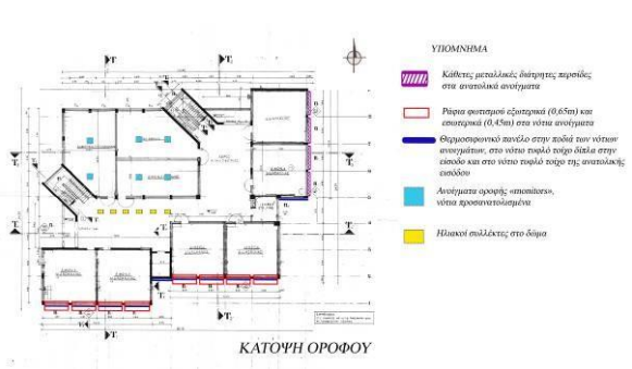
βιοκλιματικής συμπεριφοράς κάτοψη ορόφου
