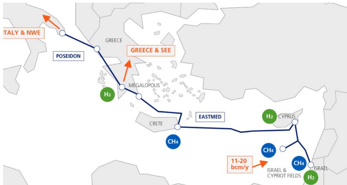
Διάγραμμα 5: EastMed Pipeline.
