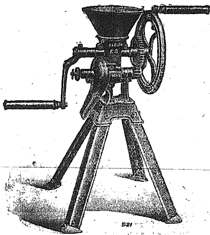
Πουργυρομηχανή χειροκίνητος άλέθει και κριθάρι, όσροβον κουκκιά και άραβόσιτον.
