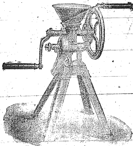
Πουργομηχανή χειροκίνητη αλέθει και κριθάρι, όρβον κοκκία και άραβόσιτον.
