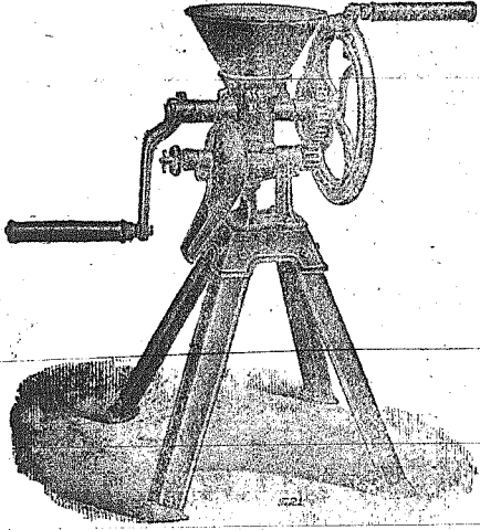
Πουργομηχανή χειροκίνητος αλέθει και κριθάρι, όροβον κουκκία και άραβόσιτον.
