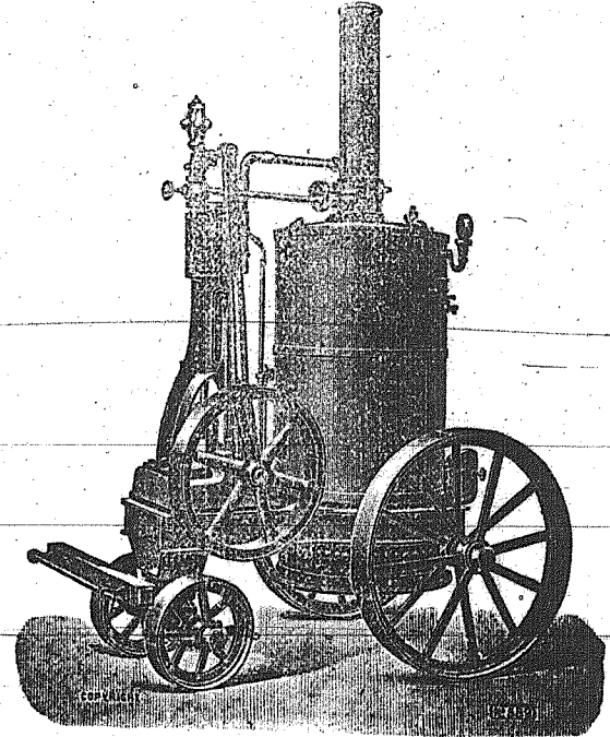
Κινητή όρθια άτμομηχανή.
