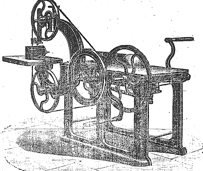
Πριονιστική μηχανή κινουμένη δια της χειρός ή με άτμην και παρέχουσα κορδέλλαν και δίσκους.
