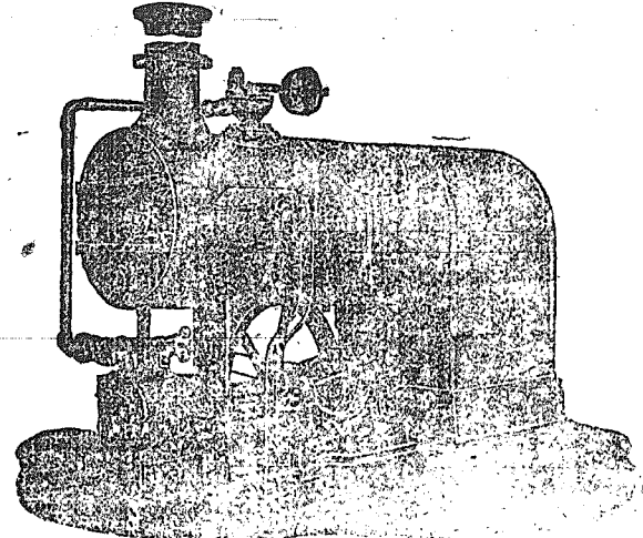
'Ατμομηχανή 6-16 ίππων με την μηχανή της τοποθετημένη κάτωτι του λέβητος παρέχουσα εύτω οικονομίαν εις την τοποθέτησιν αυτης.
