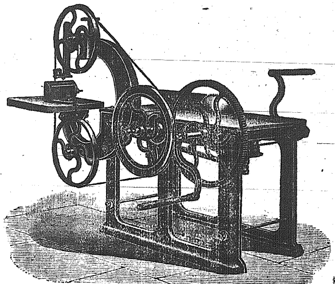
Πριονιστική μηχανή κινούμενη διά της χειρός ή με άτμον και παρέχουσα κορδέλλαν και δίσκους.
