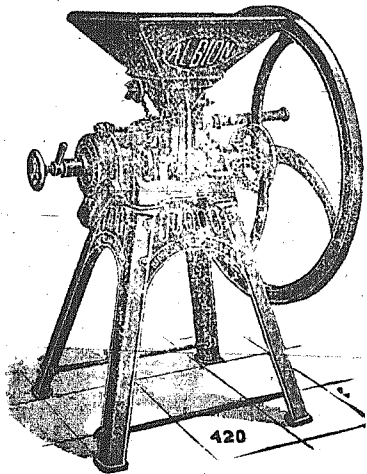
Πουργυρομηχανή χειροκίνητος αλέθουσα και κριθάρι, όροβον, κουκκιά και άραβόσιτον.
