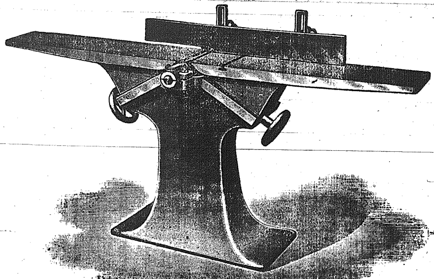
Ρυπανιστική μηχανή. — Δυνατόν να καθαίρει από τα 4 μέρη άνω των 40 νεροσανίδων την ύφαν. Άπλοῦς τοπος και εύκολος ό τρόπος.
