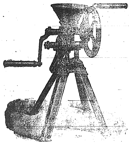
Πουργουρομηχανή χειροκίνητος ἀλφει καὶ κριθᾶρι, ὄροβον κουκκία καὶ ἀραβόσιτον.
