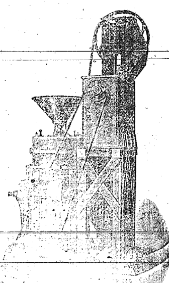
Μύλος, ἀναβιβαστήριον καὶ σημιδαίερα συννηνωμένα.
