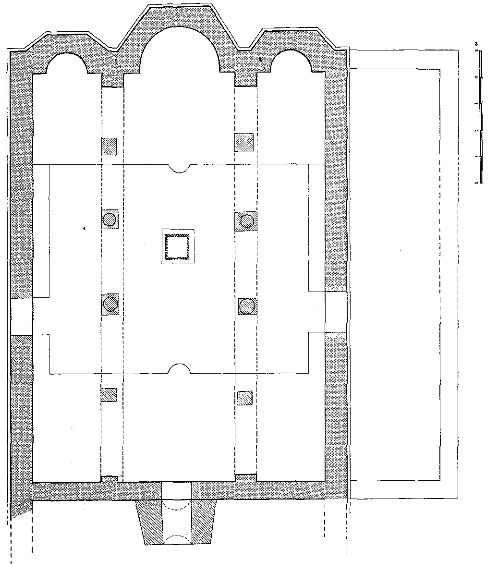
Σχέδ. 1. Άγιος Ίωάννης Δρακοσπηλιάς. Ή κάτωψη του ναού.
