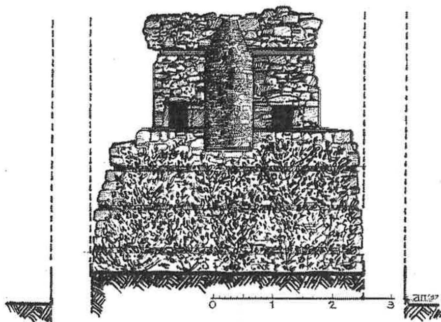
Είλκ. 15. Κτήριο Α. Έσωτερική όψη δυτικού τοίχου. Στὸν ὄροφο ἔχνη ἐστίας, οἱ δύο ἐκατέρωθεν θυρίδες καὶ —στὶς δύο ἄκρες— τὰ κατάλοιπα ἀπὸ σταθμούς («λαμπάδες») δύο παραθύρων, κάτω δὲ στὸ ἰσόγειο τρεῖς σειρὲς ξυλοδεσιές (Σχέδιο 1997)
