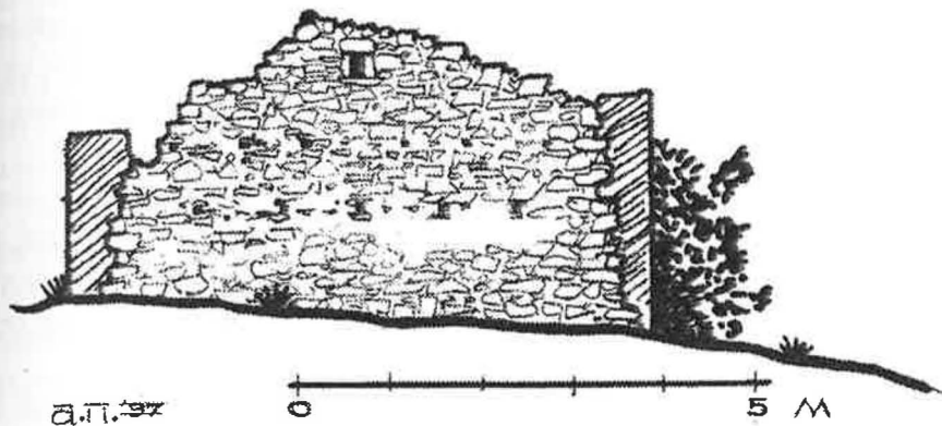
Εἰκ. 22. Κτήριο Β: Βόρεια πλευρά. Σώζεται σχεδὸν τὸ ἀρχικὸ ὕψος, διακρίνεται χοντρικὰ ἢ ἀρχικὴ, «ἀετωματικὴ» ἀπόληξή του. Οἱ γωνιόλιθοι ἔπεσαν θύματα ἀρπαγῆς, καὶ στὶς δύο (σὲ ὅλες) τὶς γωνίες (1997). Πρβ. εἰκ. 18.
