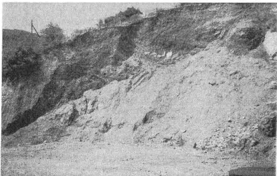
Εἰκ. 23. Χωματοληψία σὲ βάθος ἄλλαξε τὸ νότιο πρηνὲς ἐξάρματος μὲ τὸ Ὄθωμανικὸ συγκρότημα (1997)
