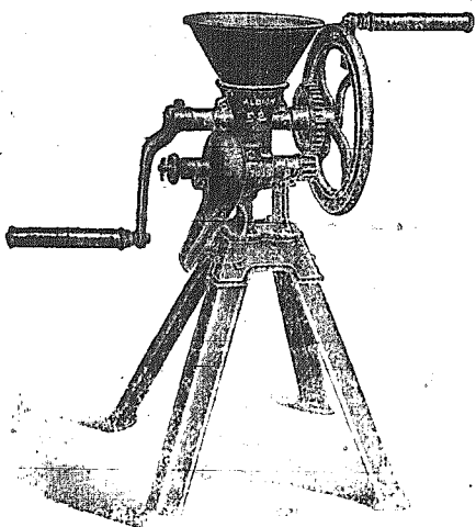
Πουργορρομηχανὴ χειροκίνητος ἀλέθει καὶ κριθάρι, ὄρεον χρονκαὶ καὶ ἀραβόσιτον.
