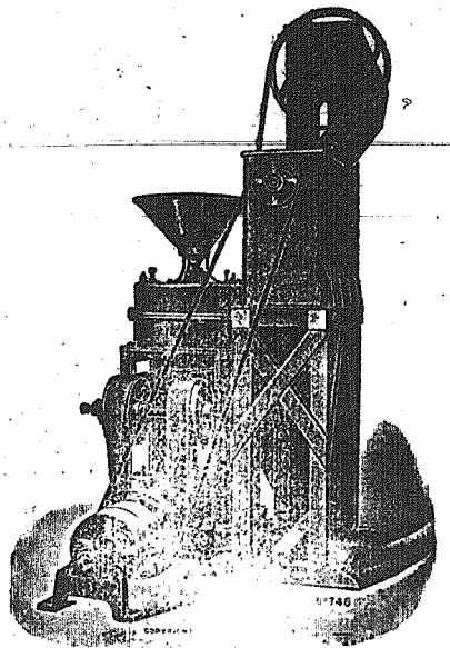
Μύλος, άναβιστήριον και σημιδαίρα συννηωμένα.
