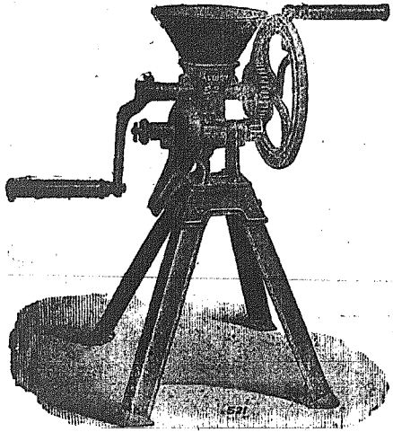
Πουργομηχανή χειροκίνητος λέβητα και κρηβάρι, δροβον κουκκιά και δαβρόστον.
