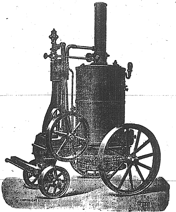
Κινητή όρβια άτμομηχανή.
