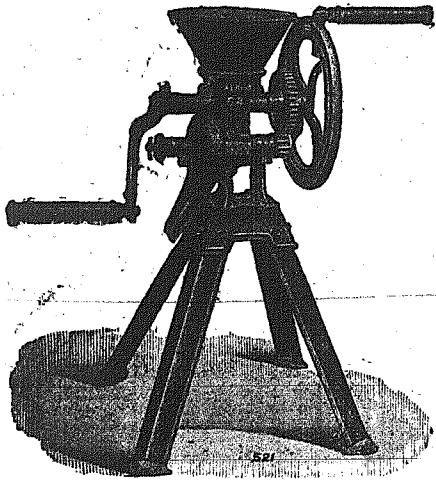
Πουργορομηχανή χειροκίνητος ἀλέθει καὶ κριθάρια, ὄρεθρον κουνικία καὶ ἀραβόσιτον.
