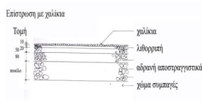
Εικόνα 5: Τομή επίστρωσης με χαλίκι
