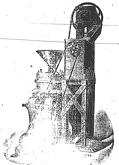
Μύλος, ἀναψιβατήριον και σημιδαλῖρα συννηωμένα.
