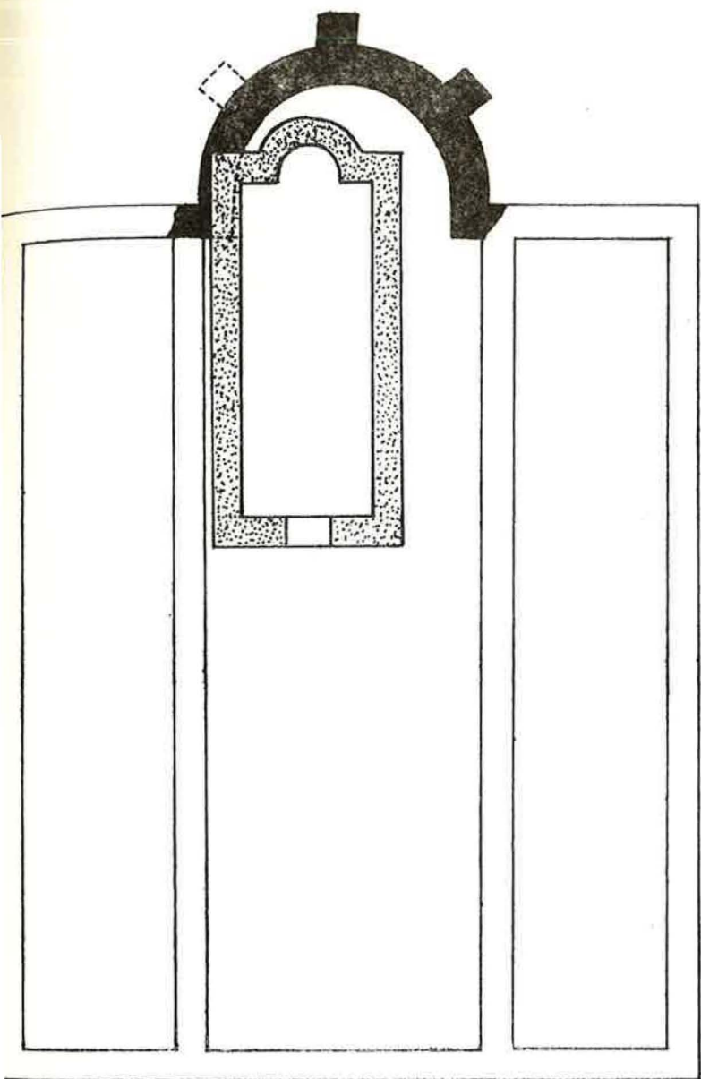
Σχέδ. 5. Κάτοψη τῆς βασιλικῆς τοῦ λόφου Ἁγ. Ἰωάννης κοντὰ στὴ Γουριὰ.
