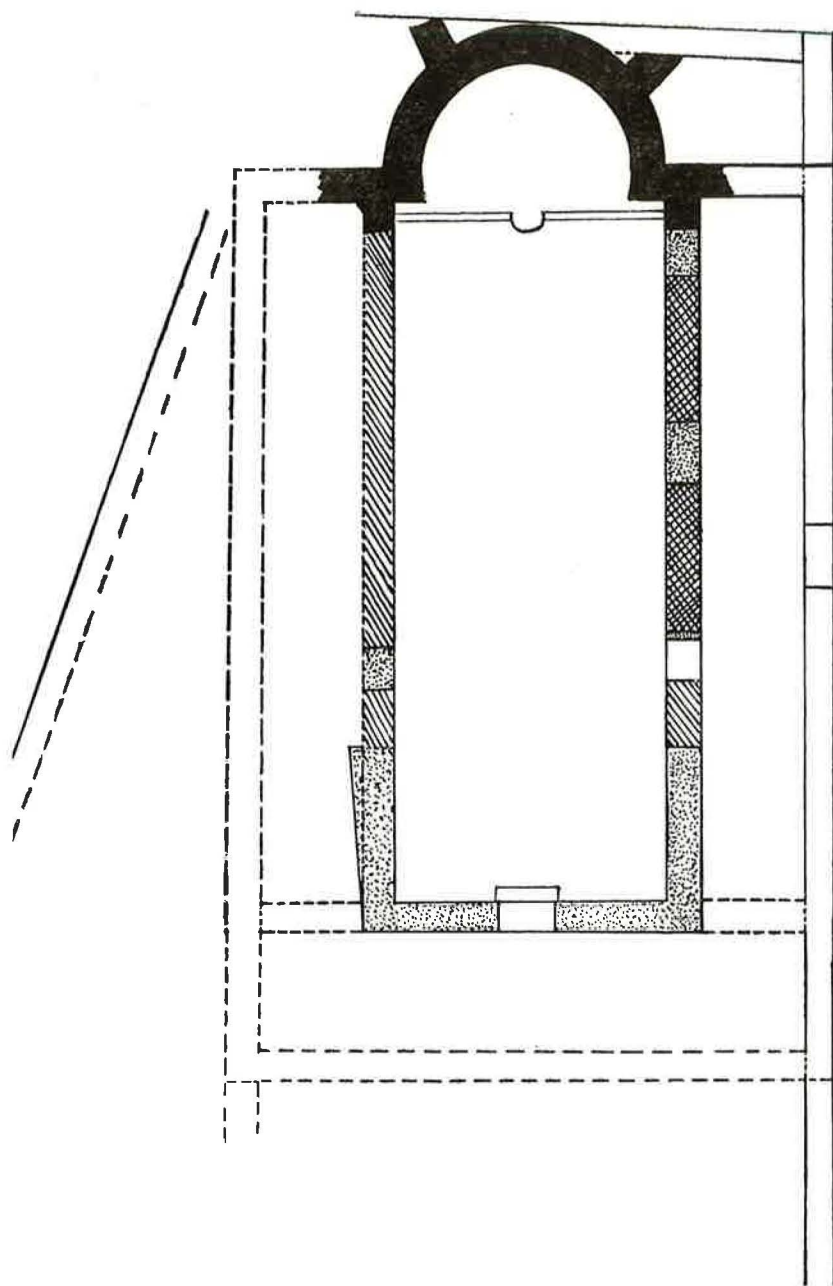
Σχέδ. 6. Κάτοψη τῆς βασιλικῆς τῆς Παραφράς.
