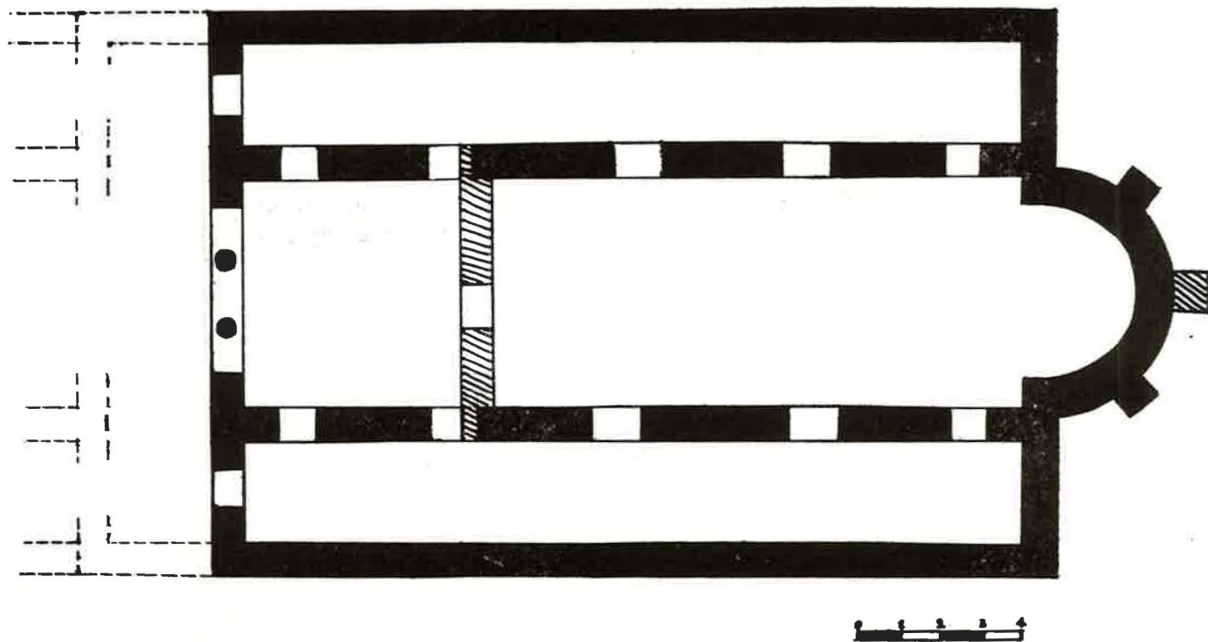
Σχέδ. 2. Κάτοψη τῆς βασιλικῆς τοῦ Ἁγ. Γεωργίου Εὐηνοχωρίου (πρόταση γιὰ τὴν ἀποκατάσταση τοῦ σχεδίου).
