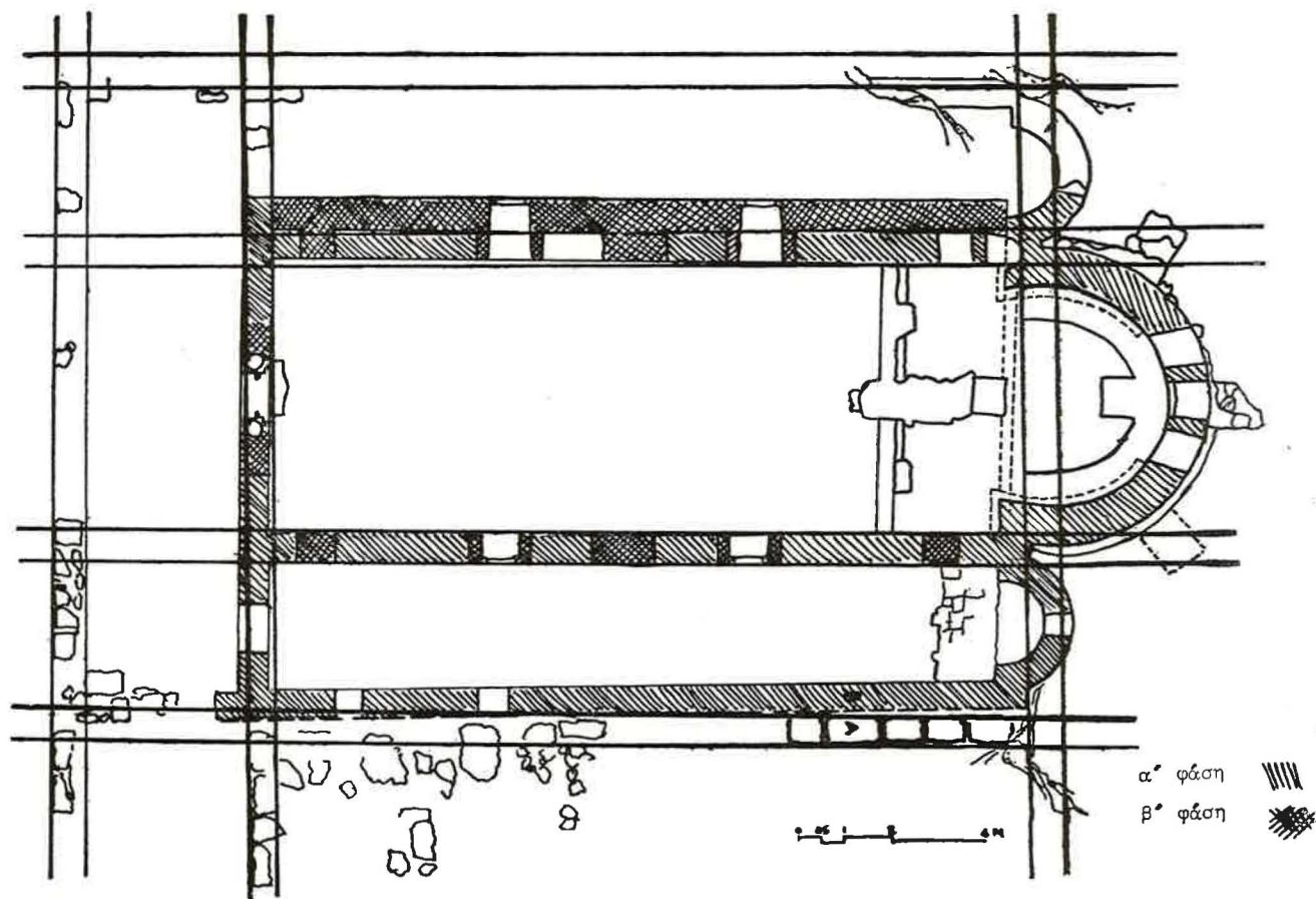
Σχέδ. 4. Κάτοψη της βασιλικής της Μάστρου (προηγούμενο σχέδιο): πρόταση για τη χάραξη του κανάβου.
