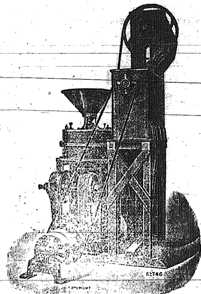
Μύλος, ἀναβιβαστήριον καὶ σημιδαλέρα συννηωμένα.
