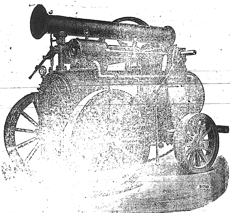
Κινητὴ ἀτμομηχανὴ μὲ ἓνα κύλινδρον.
