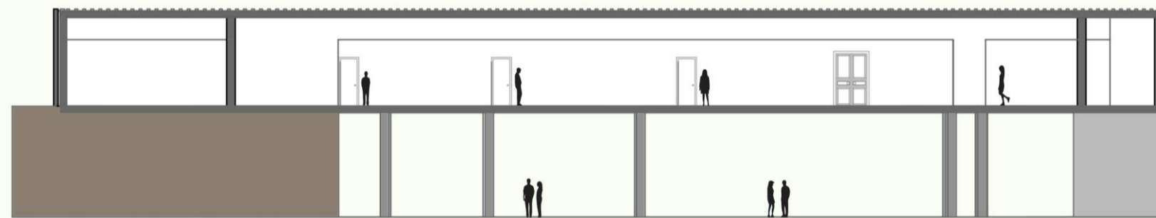
SECTION A-A
