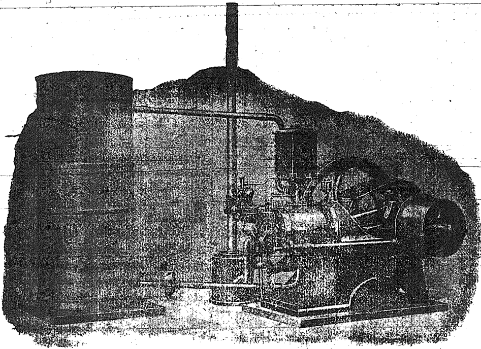
Πετρελαιομηχανή με αποθήκην ύδατος.
