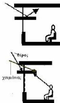
Σχ. Ηλιακά ράφια (Πηγή: www.energysmartschools.gov )
