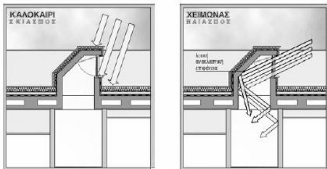
Σχ. Άμεσο ηλιακό κέρδος από τα νότια ανοίγματα στην οροφή. Χειμερινή και θερινή λειτουργία.
