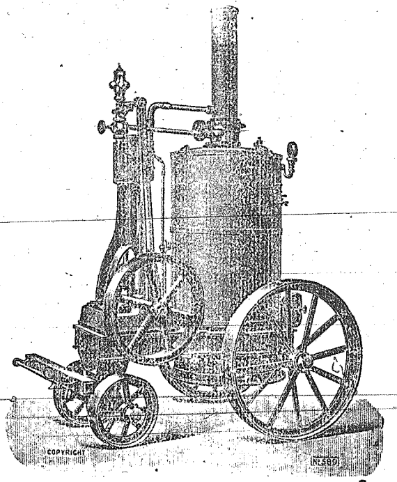
Κινητή θορία άτμομηχανή.
