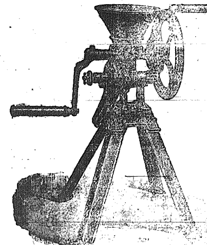
Πουργορομηχανή χειροκίνητος ἄλθει καὶ κριθᾶρι, ὄροβον κοσκίδια καὶ ἀραβόσιτον.
