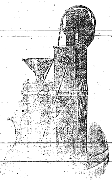
Μύλος, ἀναβιβαστήριον καὶ σημιδαλέρα συννηωμένα.
