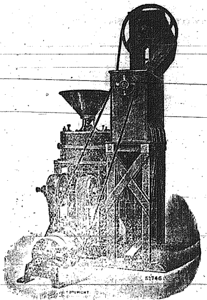
Μύλος, ἀναβιβαστήριον καὶ σημιδαλέρα συνηλωμένα.
