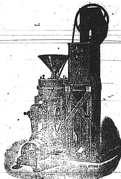
Μύλος, άναβιβαστήριο και σημιδαλέρα συννηωμένα.
