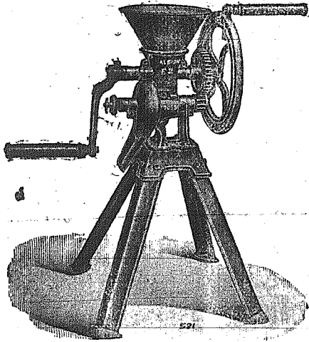
Πουργομοχάνη χειροκίνητος άλεθει και κριθάρι, όρβορον κοουκιά και άραβόκοιτο.
