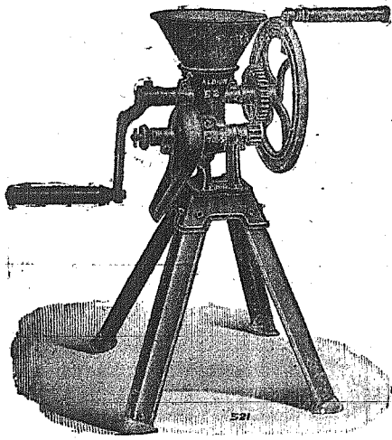
Πουργομηχανή χειροκίνητος άλεσται και κριθάρι, όροβου, κουκκιά και άραβόστον.
