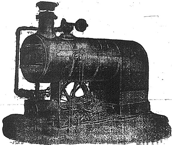
Ατμομηχανή 6—16 ίππων με την μηχανή της τοποθετημένη κάτω του λέβητος παρέχουσα ζούτα οικονομίας εις την τοποθέτησιν αυτής.
