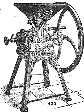
Πουργούραμηχανή χειροκίνητος αλέθουσα και κριθάρι, έρβον, κόκκια και άραβόσιτον.
