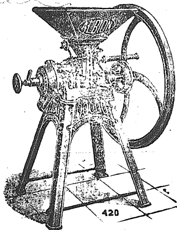
Πουργυρομηχανή χειροκίνητος αλέθουσα καφέ, κριθάρι, όροβον, κουκκία και άρβουσιτον.
