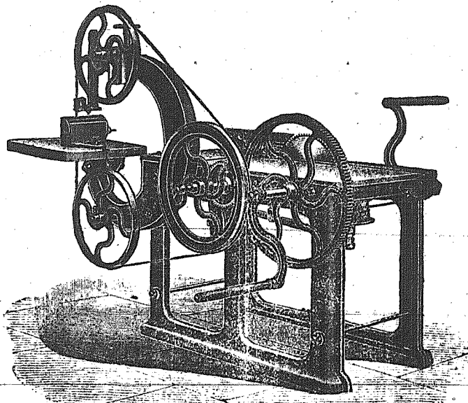
Πριονιστική μηχανή κινουμένη, δια της χειρός ή με άτμων και παρέχουσα κορδέλλαν και δίσκους.
