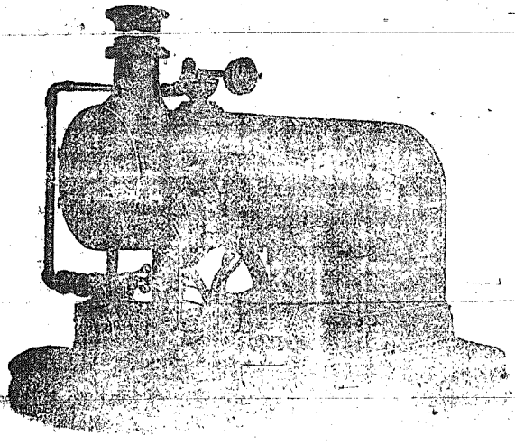
Ατμομηχανή 6-16 ίππων με την μηχανή της τοποθετημένη κάτω τοι λείψτος παρέχουσα ούτω οικονομίαν εις την τοποθέτησιν αυτής.
