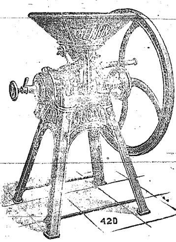
Παυρομηχανή χειροκίνητος ελέφουσα και κοιλίρι, όροβον, κουκκιά και άραβόσιτον.
