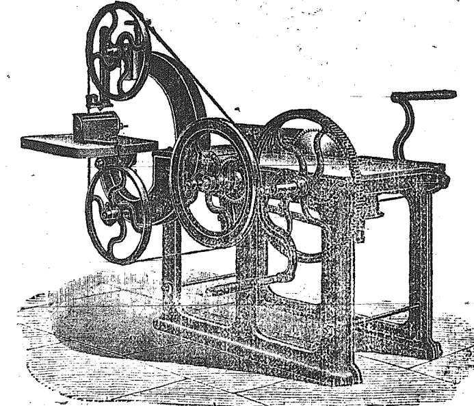
Πριονιστική μηχανή βινουμένη διά της χειρός ή με άτμων και παρέχουσα κερδέλλαν και δίσκου.
