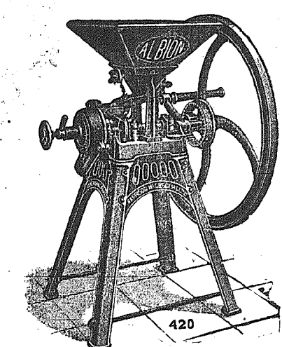
Πουργυρομηχανή χειροκίνητος αλέθουσα και κριθάρι, όρβον, κουκκιά και άραβόσιτον.
