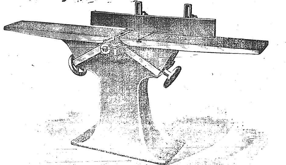
Ροκανιστική μηχανή.— Δύναται να ροκανίση από τά 4 μέρη άνω των 40 νεροσανίδων την ύραν. Άπλούστατος και εύκολος ο τρόπος.
