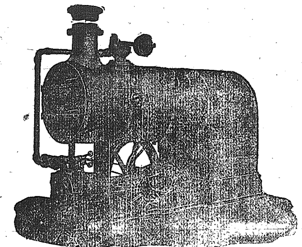
Ατμομηχανή 6—16 ίππων με την μηχανή της τοπο- θετημένη κάτωθι του λέβητος παρέχουσα ούτω οικονο- μίαν εις την τοποθέτησιν αυτής.
